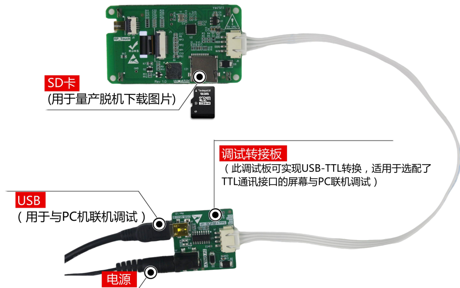
图 1-4 调试工具图
