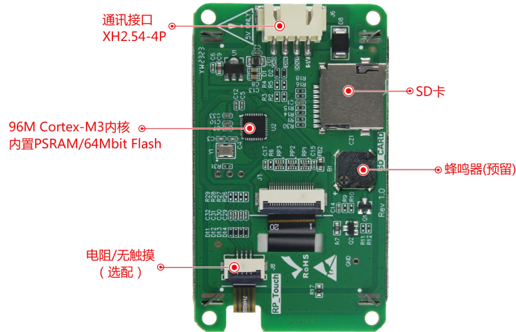
图 1-3 硬件配置图
